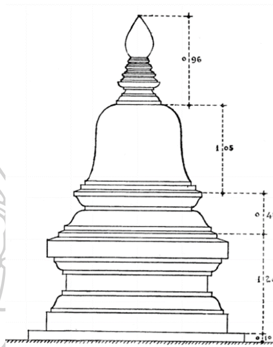
ภาพที่ 49: ภาพลายเส้นของเจดีย์ทรงระฆังที่ วัดเทพพนม จังหวัดเสียมเรียบ 93
